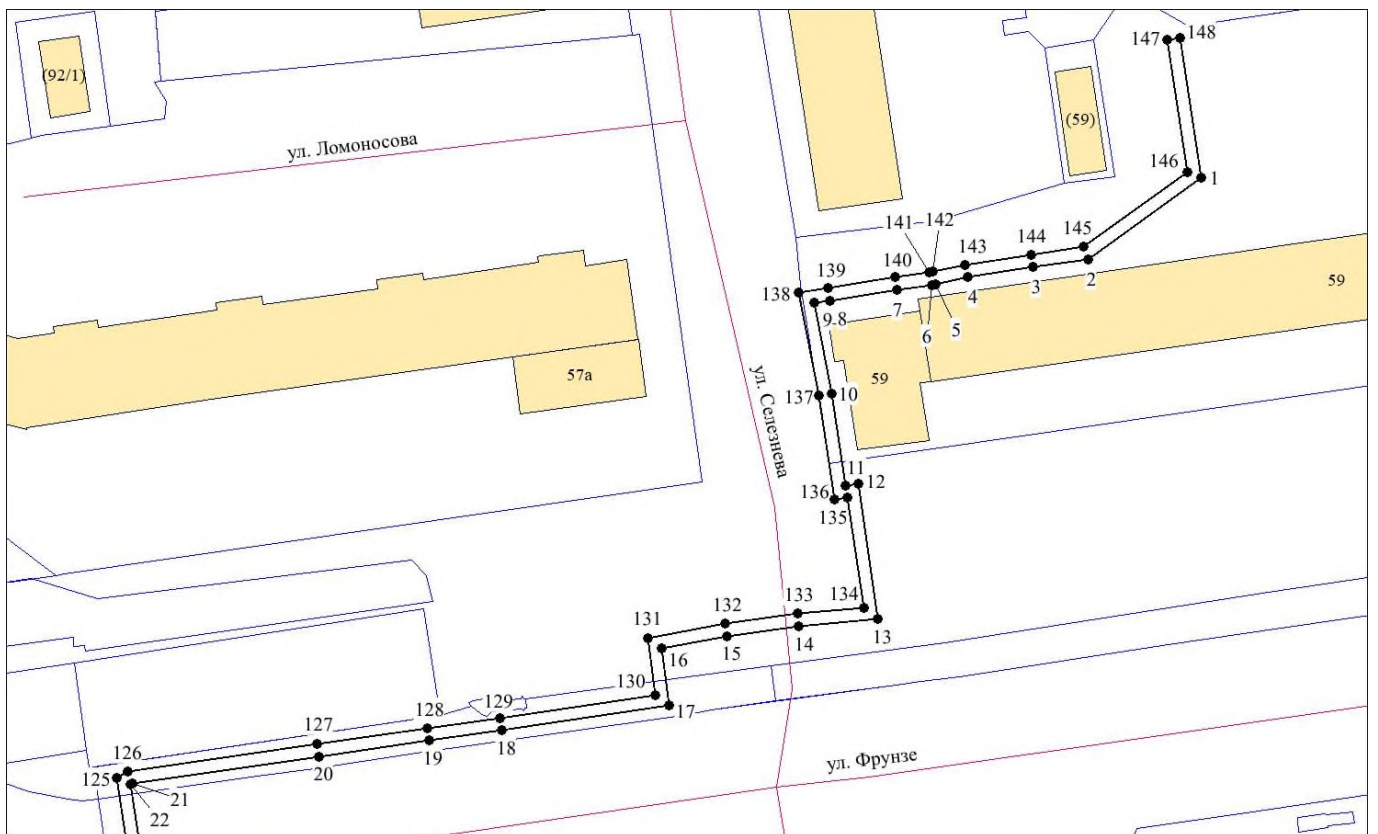
Выносной лист 1
